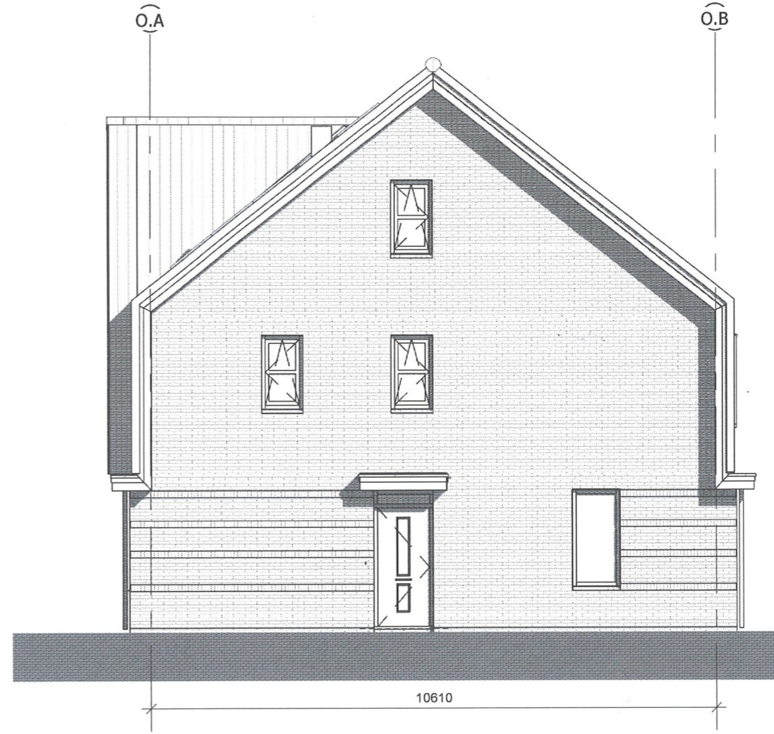
rechter zijgevel
