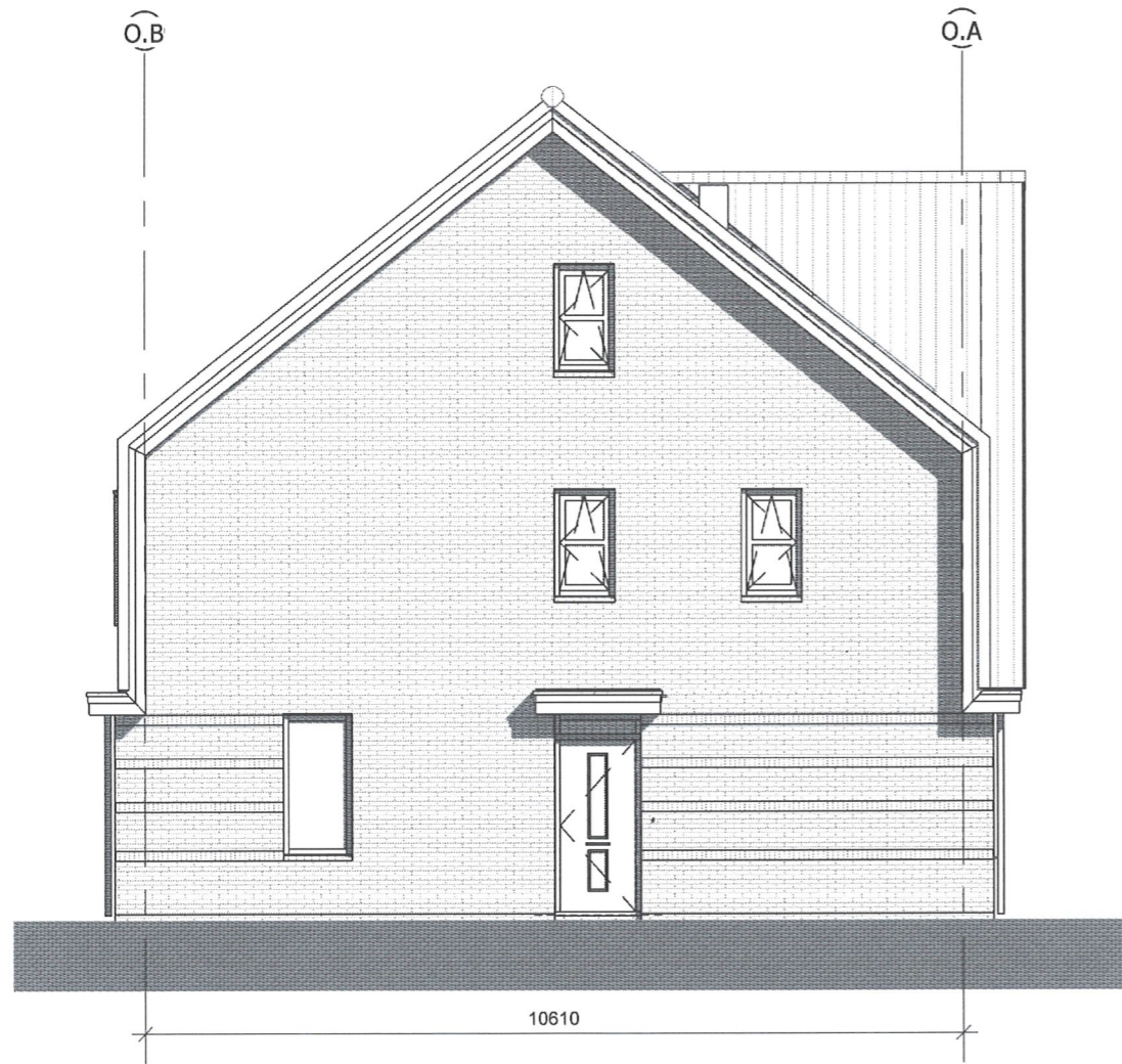
linker zijgevel
